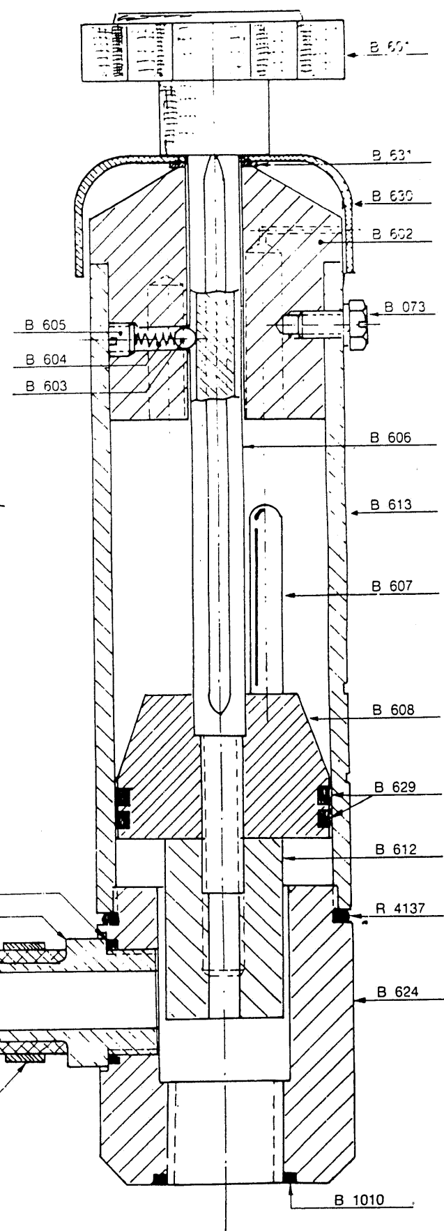
INJECTEUR KOMPLEET B 600
